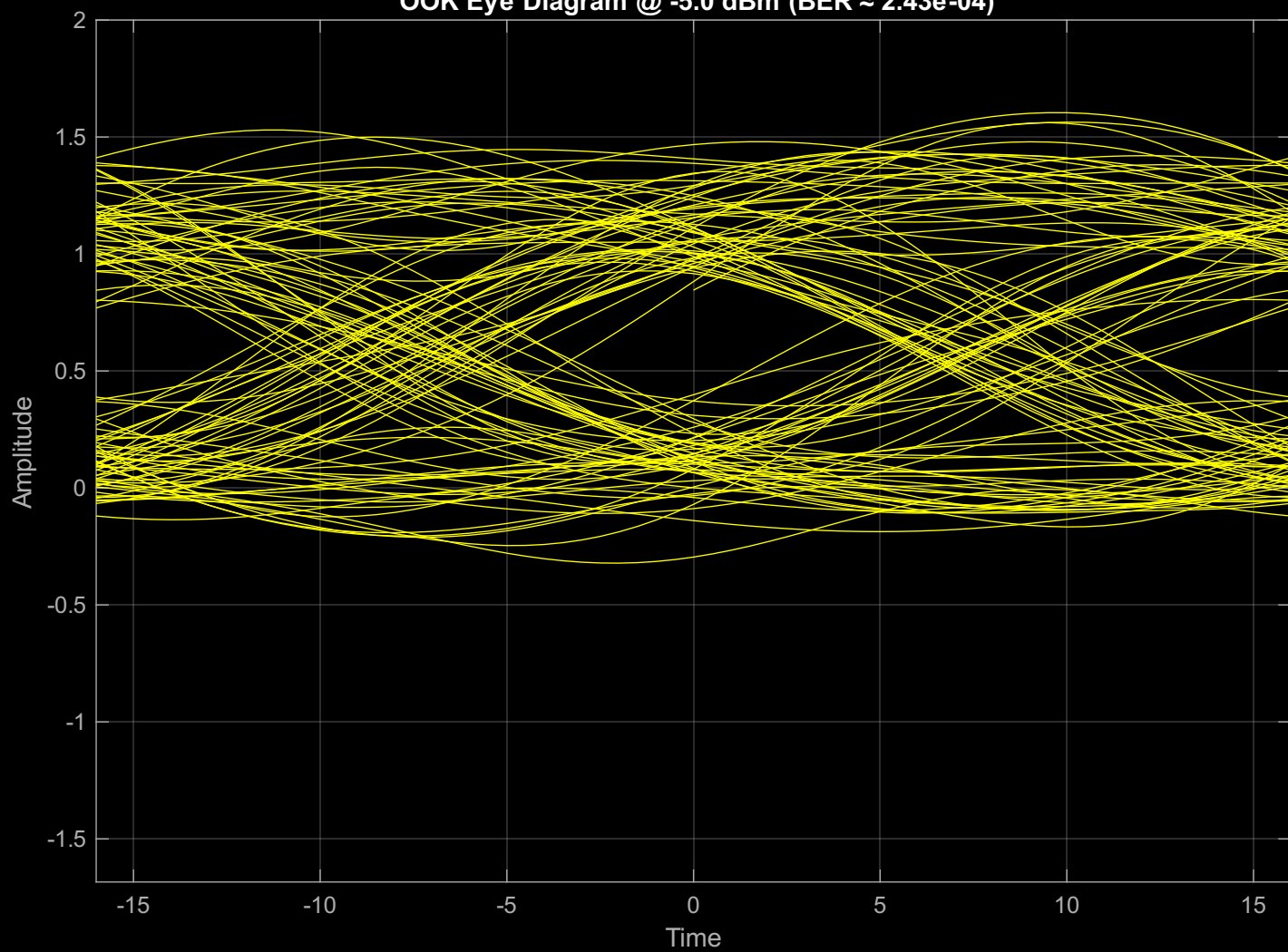
OOK Eye Diagram @ -5.0 dBm (BER \approx 2.43\text{e-}04 )
